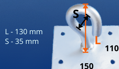
hak płytowy na ścianę, ocynk
