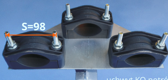
uchwyt KO potrójny, słup EPV rozmiar 75, ocynk
