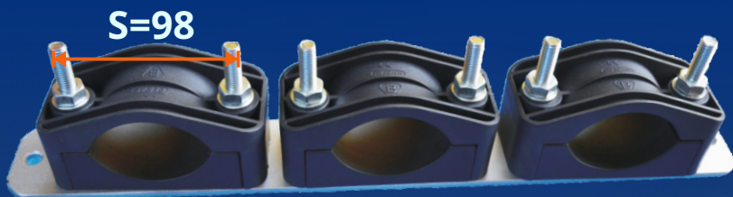
uchwyt KO potrójny, na listwie rozmiar 75, ocynk
