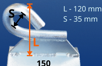
hak płytowy O18 na słupy EPV, ocynk
