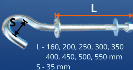
uchwyt oczkowy M16, ocynk
